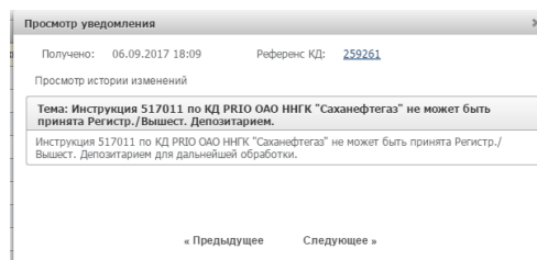
Рисунок 17. Просмотр уведомления
