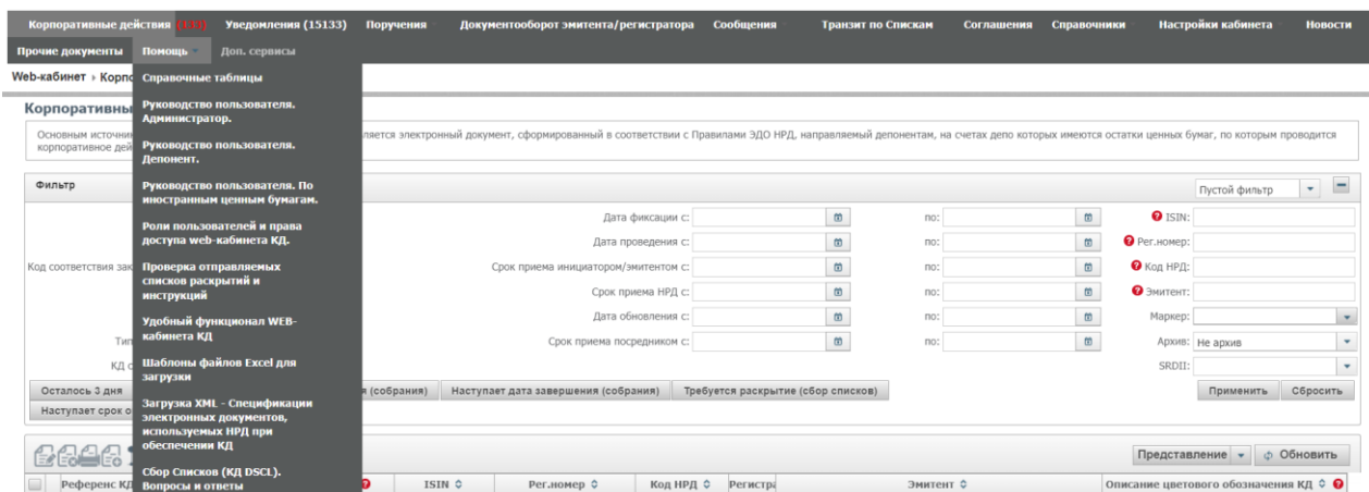
Рисунок 273. Раздел «Помощь»
