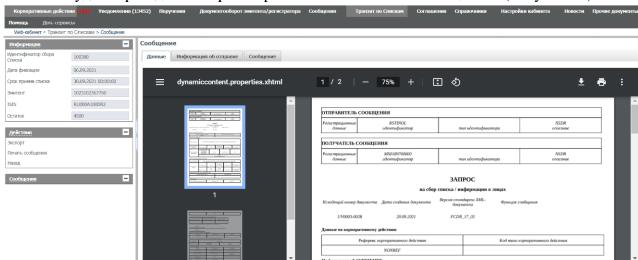
Рисунок 26. Форма «Сообщение»
