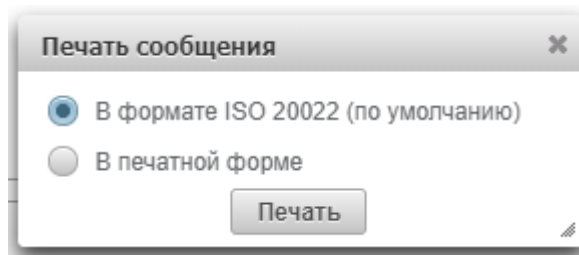
Рисунок 258. Печать сообщения
